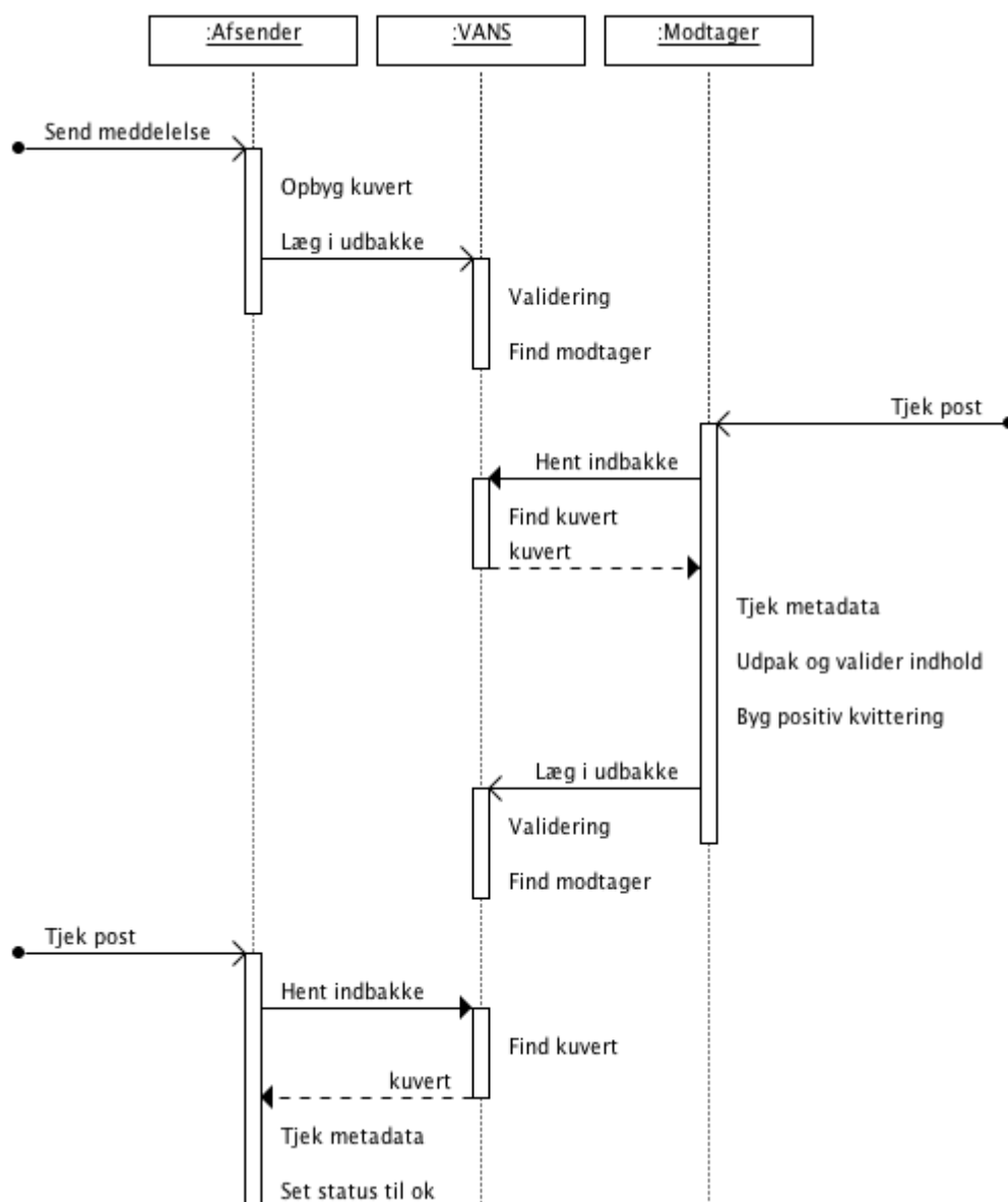
Figur 2.1. Sekvensdiagram
